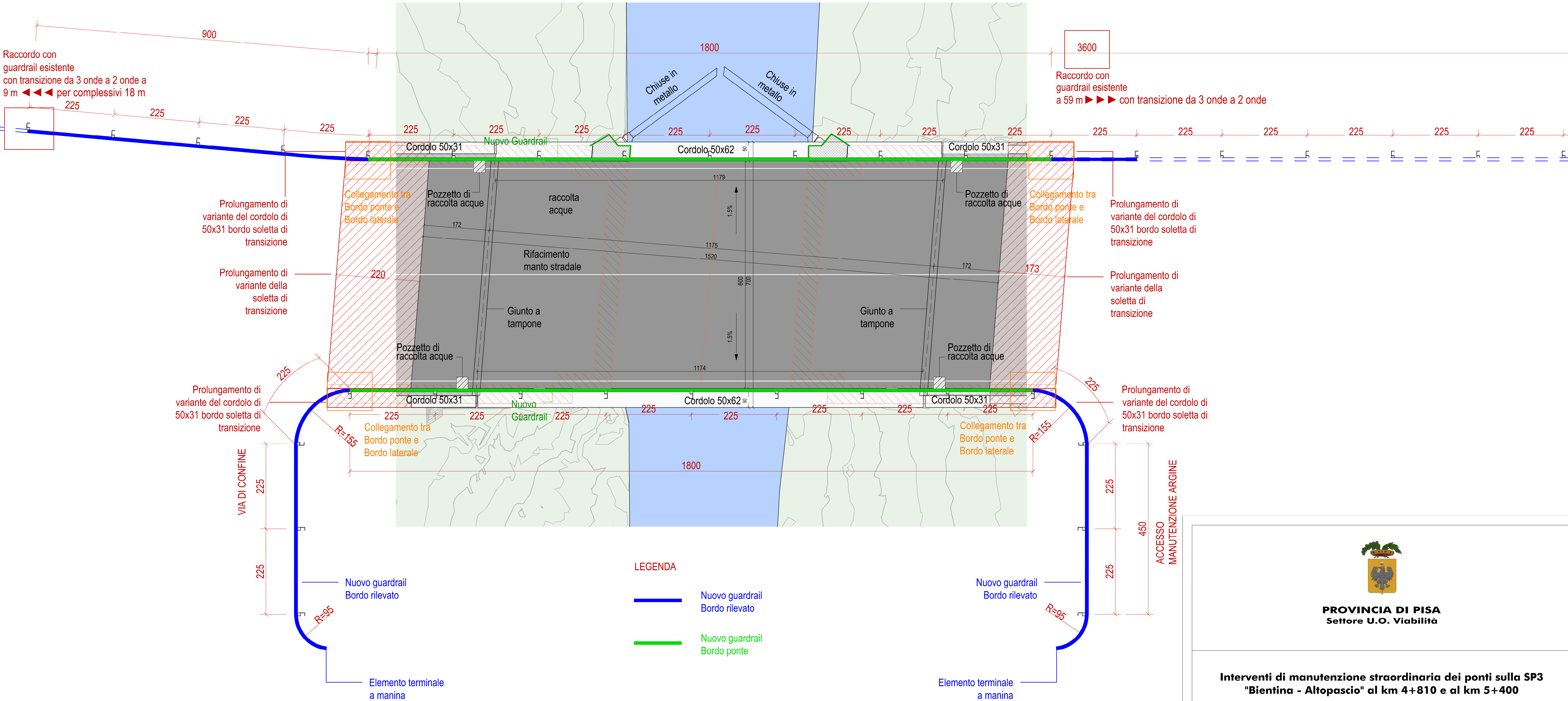
PIANTA | IMPALCATO STRUTTURALE, PALI DI FONDAZIONE E PROLUNGAMENTO SOLETTE DI TRANSIZIONE
